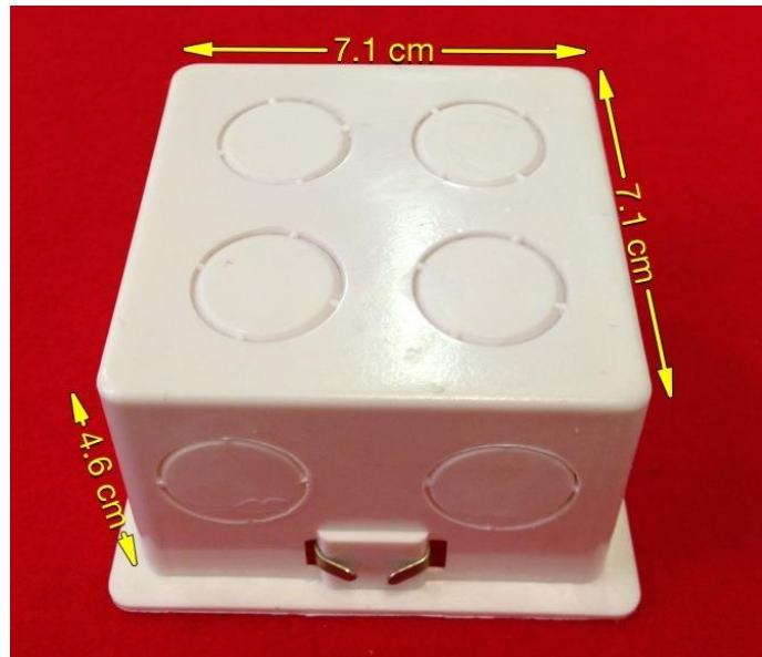
Scatola per incasso nel muro
